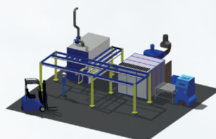
Cabine de grenaillage / sablage
