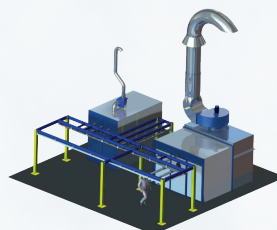
Cabine de peinture liquide
